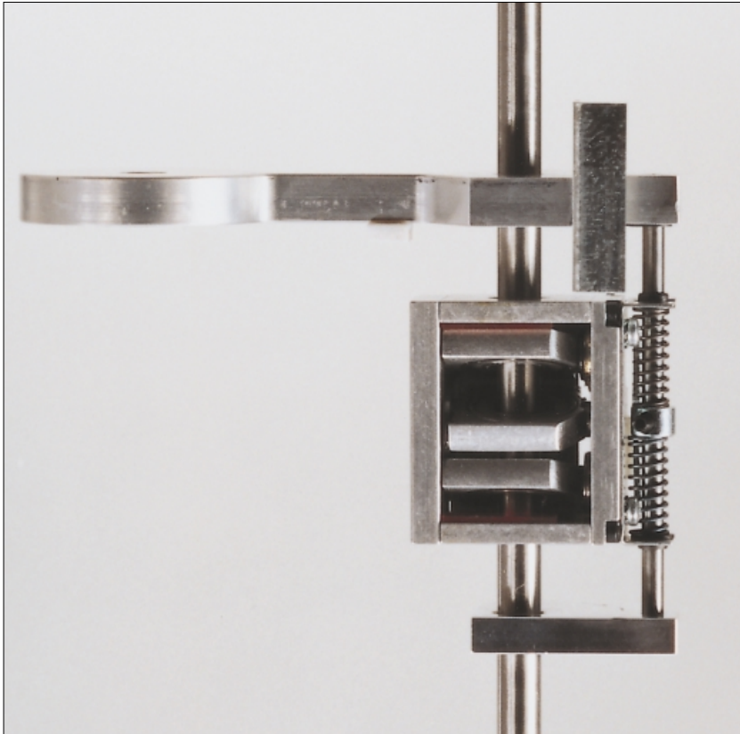
Hubgetriebe RG 3-12-OMX / Traversing Drive RG 3-12-OMX
